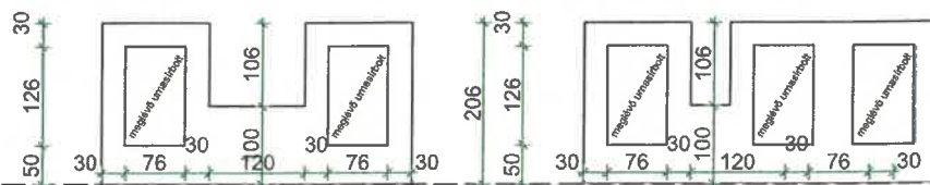
Meglévő sírhelyek környezetének burkolása. Tervezett burkolat nagysága: 8,5 m 2 , 22 fm kerti szegéllyel
